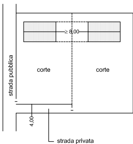
modulo binato
