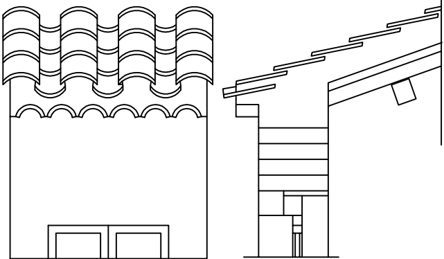
aggetto con filare di coppi annegati nel cordolo
