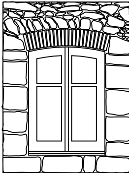
apertura con arco di scarico in laterizi
