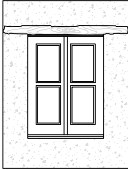
apertura elementare con architrave ligneo
